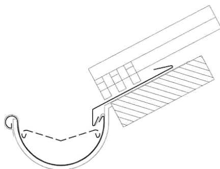
Odkap z odkapno pločevino
