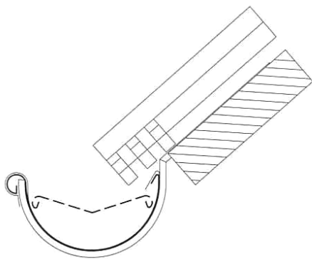
Odkap s prosto visečim strešnim žlebom
