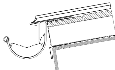
Odkap za streho z dvojnimi stojčim zgibom/letvenim sistemom
