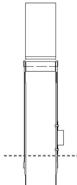
Priključek z RHEINZINK®-revizijskim pomičnim elementom
